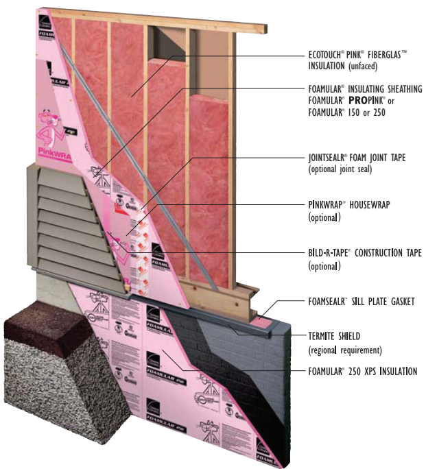
Wood Stud Framing
